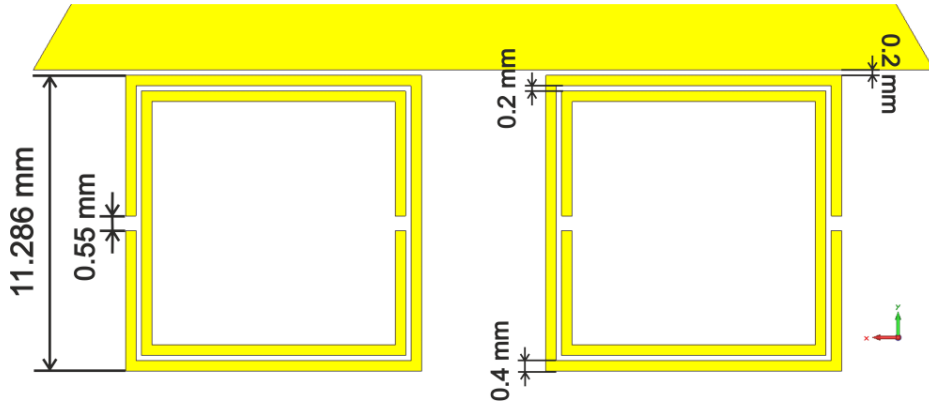
Figura 3.26 Dimensiones de los anillos optimizados a la frecuencia de 2.4 GHz. Elaborada por el Autor
