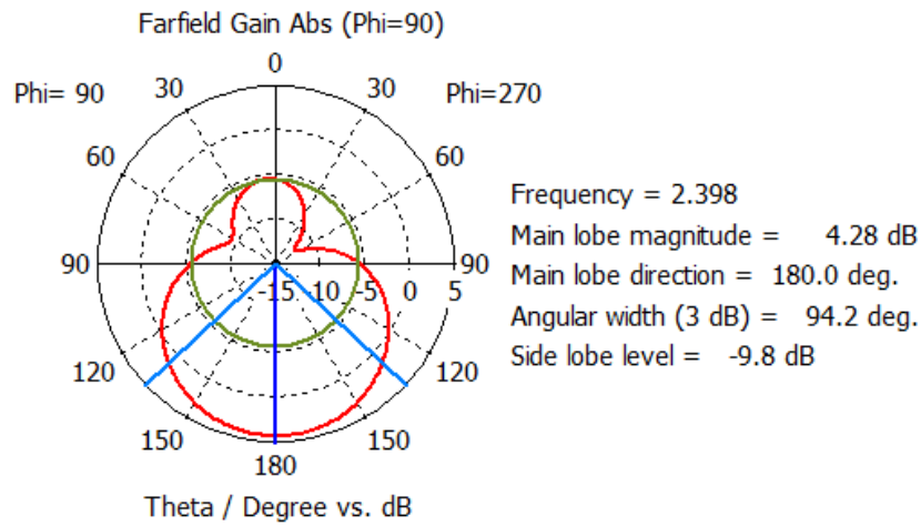
Figura 3.18 Patrón de radiación de la antena triangular alimentada por proximidad en coordenadas polares. Elaborada por el Autor
