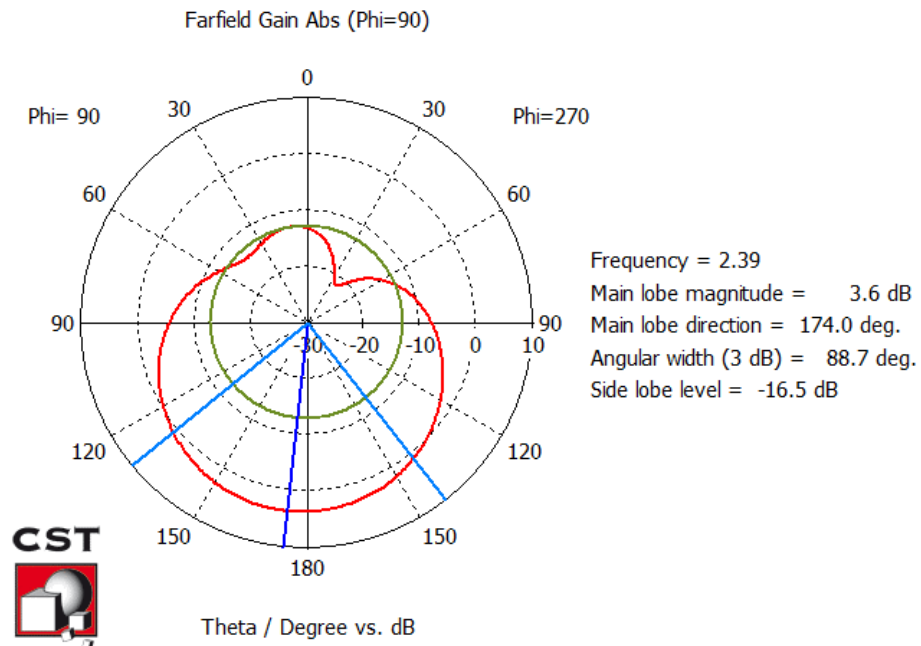
Figura 3.30 Patrón de radiación en coordenadas polares de la antena de parche triangular doble banda alimentada por proximidad a 2.39 GHz. Elaborada por el Autor
