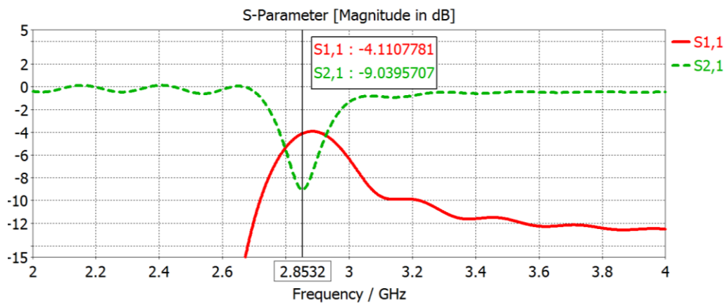
Figura 3.21 Comportamiento de los parámetros S_{11} y S_{21} para el filtro supresor de banda con dimensiones teóricas de los SRR.
