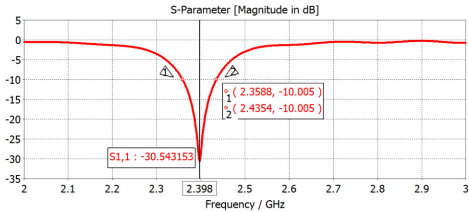
Figura 3.15 Pérdidas de retorno de la antena alimentada por proximidad optimizada ( a=35.6\text{mm} ). Elaborada por el Autor
