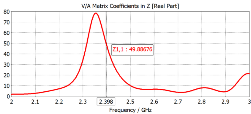
Figura 3.16 Parte real de la impedancia de entrada de la antena alimentada por proximidad optimizada ( a=35.6\text{mm} ). Elaborada por el Autor
