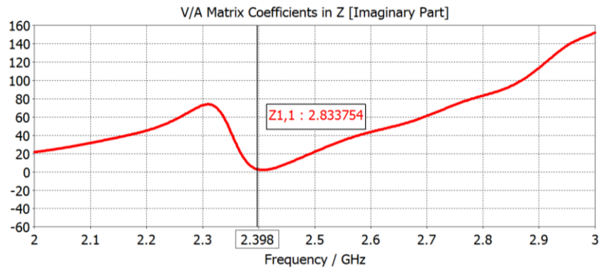
Figura 3.17 Parte imaginaria de la impedancia de entrada de la antena alimentada por proximidad optimizada ( a=35.6\text{mm} ). Elaborada por el Autor
