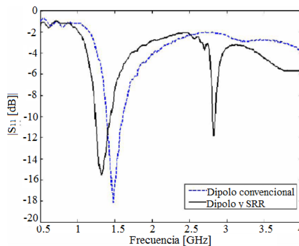
Figura 2.23 Pérdidas de retorno de la antena cargada con SRR Fuente: (Herraiz, 2010).
