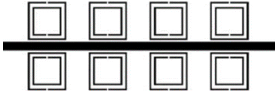
Figura 2.17 Línea de transmisión de microcintas cargada con SRR para obtener \mu_{eff} negativa Fuente: (Marqués, Martín, & Sorolla, 2008).
