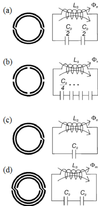
Figura 2.8 Estructuras derivadas del SRR: NB-SRR (a), D-SRR (b), SR (c), D-SR (d) Fuente: (Baena, y otros, 2005).
