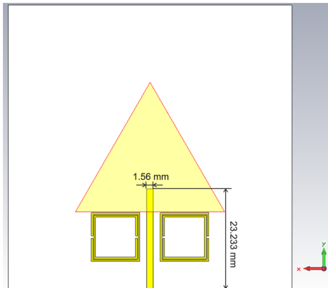
Figura 3.25 SRR acoplados a la línea de transmisión para aumentar las pérdidas de retorno a 2.4 Ghz. Elaborada por el Autor
