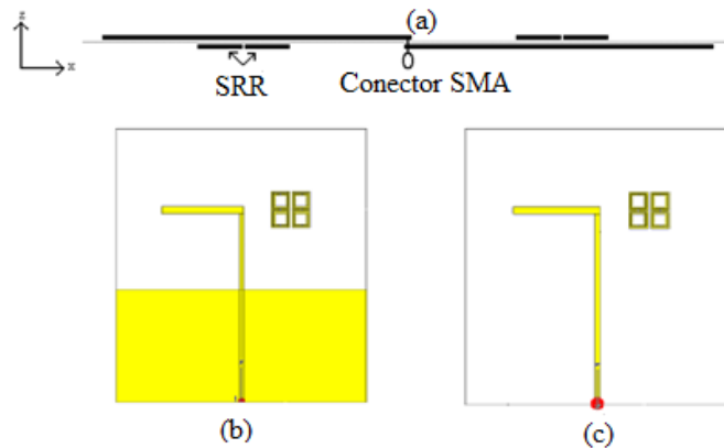
Figura 2.22 Esquema de una antena cargada con SRR: vista transversal (a), vista inferior (b) y vista superior (c) Fuente: (Herraiz, 2010).
