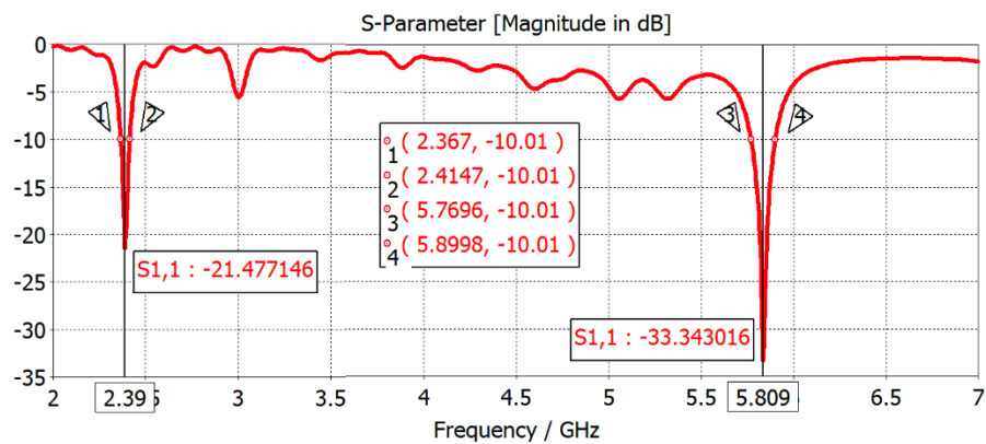
Figura 3.27 Pérdidas de retorno de la antena de parche triangular doble banda alimentada por proximidad optimizada. Elaborada por el Autor
