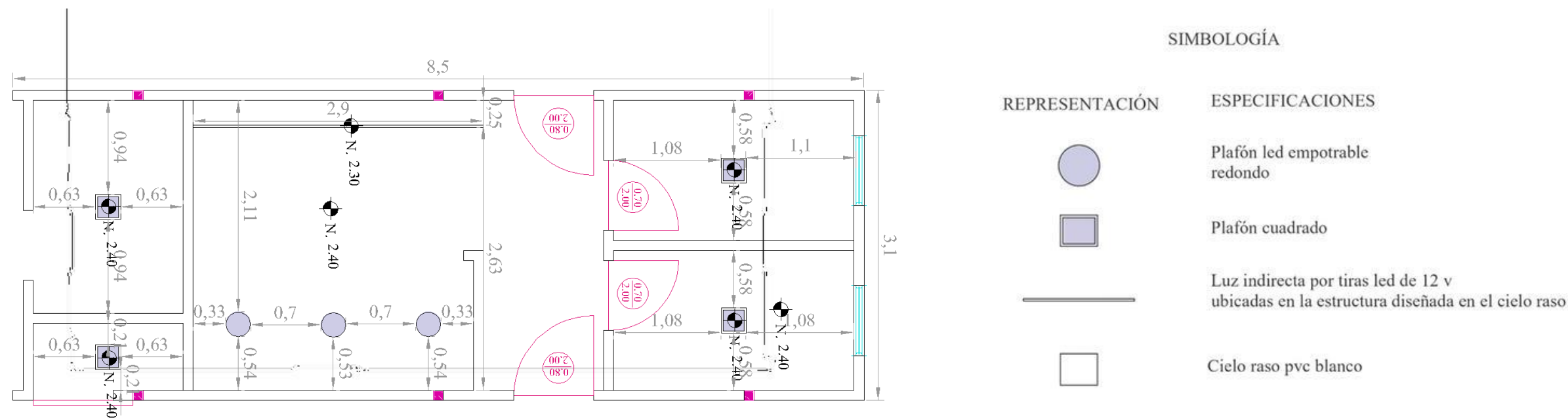
Figura 51 Plano de cielo raso y luminarias
