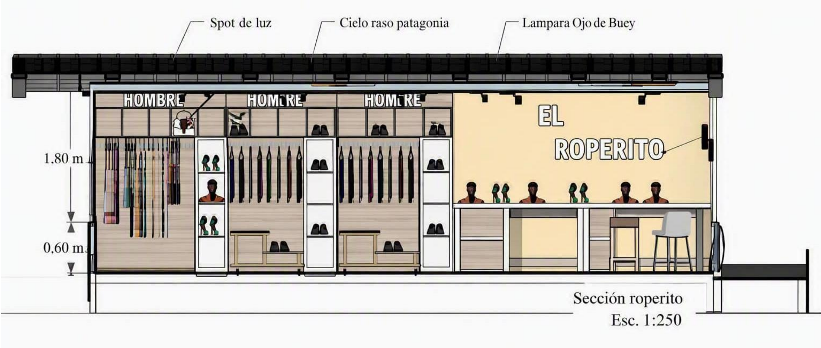
Sección roperito
