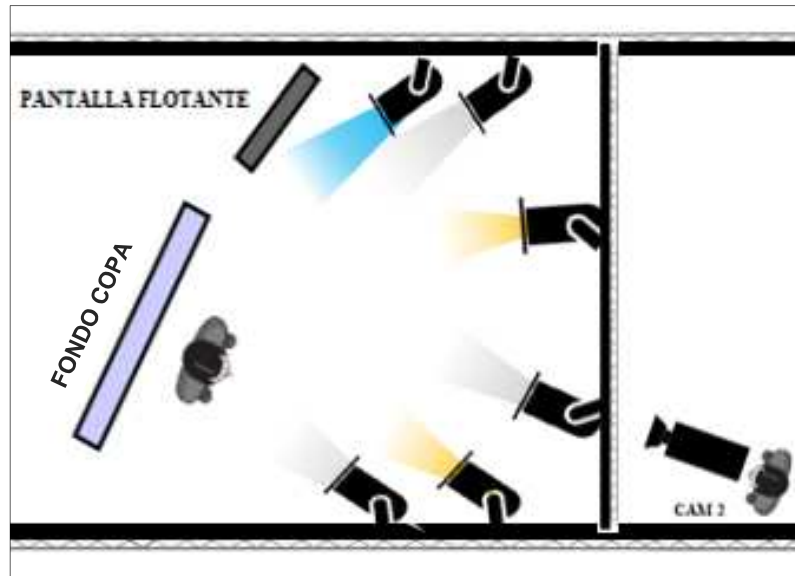
Ilustración 19 Diagrama de Planta - Set de Deportes
