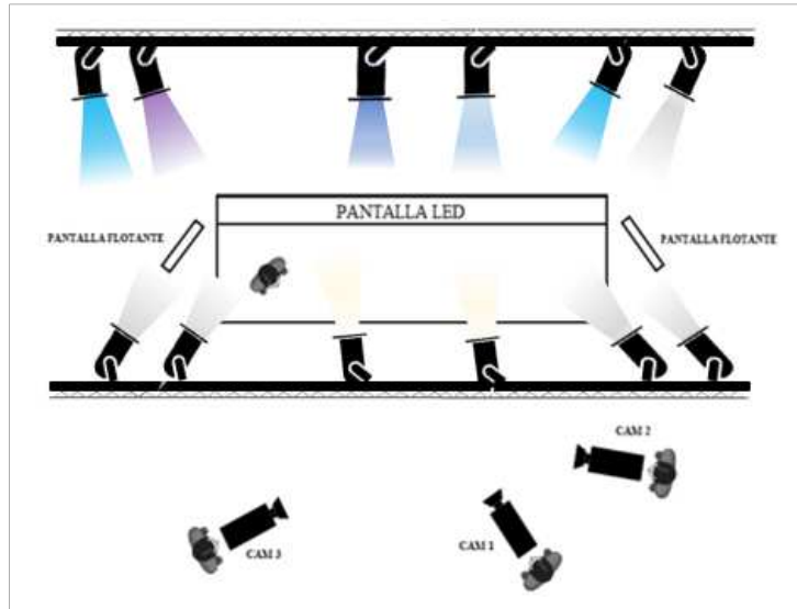
Ilustración 17 Diagrama de Planta - Iluminación Set Principal
