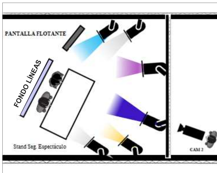
Ilustración 18 Diagrama de Planta - Iluminación Set Espectáculo
