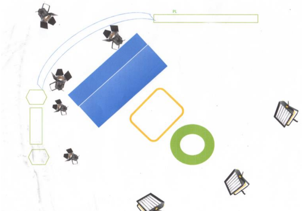
Gráfico 4 ESQUEMA DEL PLAN DE ILUMINACIÓN DEL PROGRAMA
